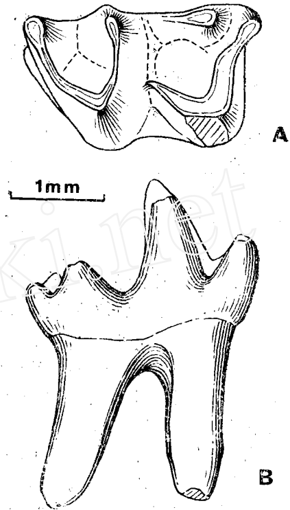
图 2 云南原细尾鼯(新属、新种),左 M_2 (V8282.13)。A,冠面视; B,舌侧视 Fig. 2 Prodendrogale yunnanica gen. et sp. nov., left M_2 (V8282.13). A, occlusal view; B, lingual view
