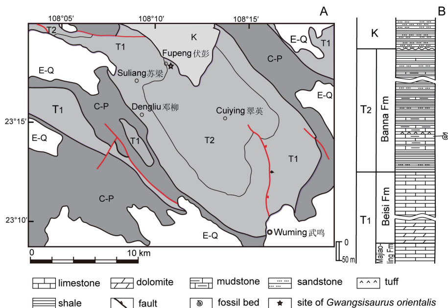
图1 广西武鸣地区地质简图及东方广西龙产地(A)和地层柱状图及化石层位(B)
