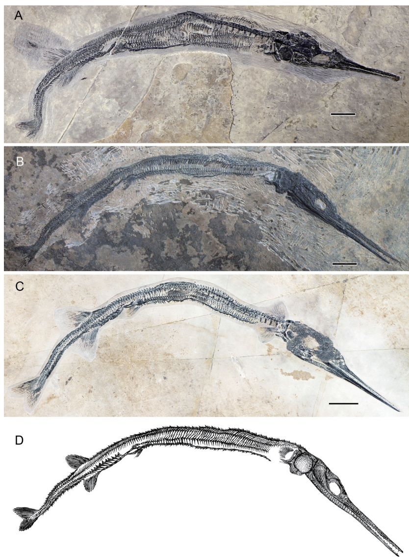
Fig. 2 Photographs (A–C) and tentative restoration (D) of Saurichthys spinosa sp. nov. A. IVPP V 23062 (holotype); B. GMPKU-P-1533; C. V 22832. Scale bars=5 mm
