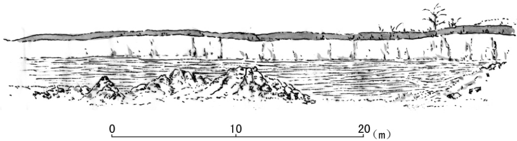
图5 阎家岗遗址沉积剖面素描图
