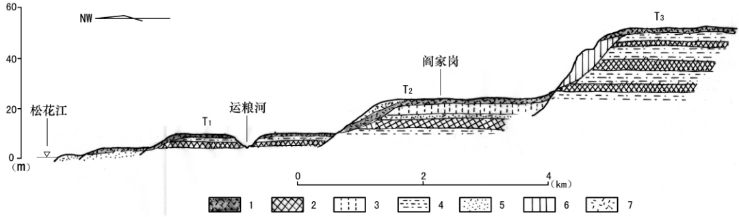
图 3 阎家岗一带松花江阶地剖面图
