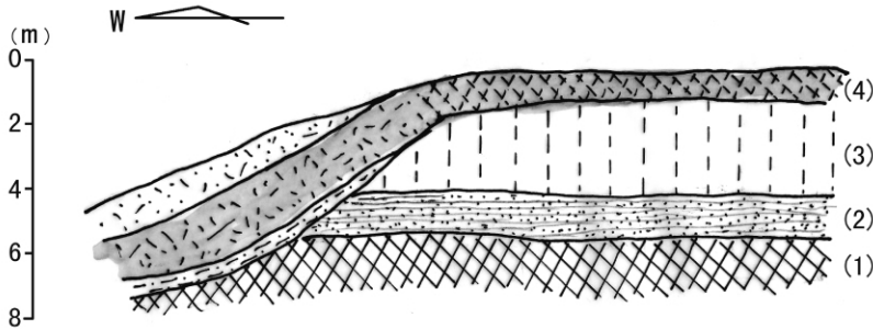
图 4 宋家店砖瓦厂剖面
