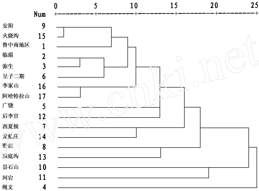
图 1 聚类分析系统树图
