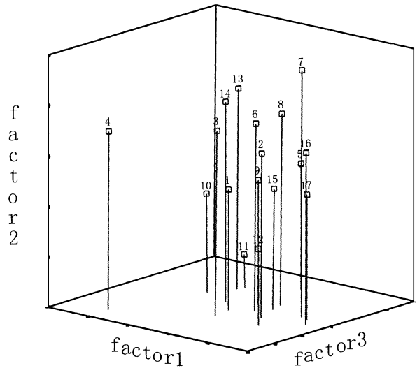
图 2 前 3 个主成分的三维坐标图
