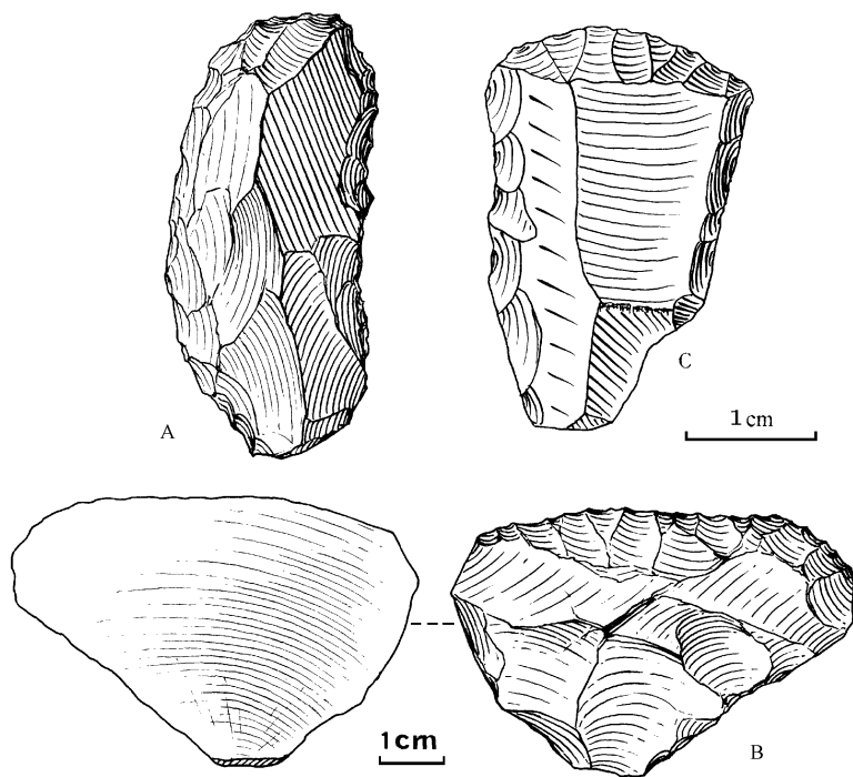
图 4 端刃刮削器 (End scrapers)
