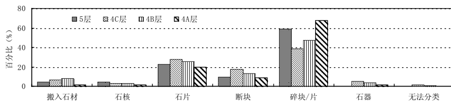
图 9 徐家城遗址各层石制品类型对比图
