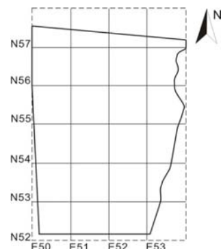
图 3 徐家城遗址发掘区探方分布图
