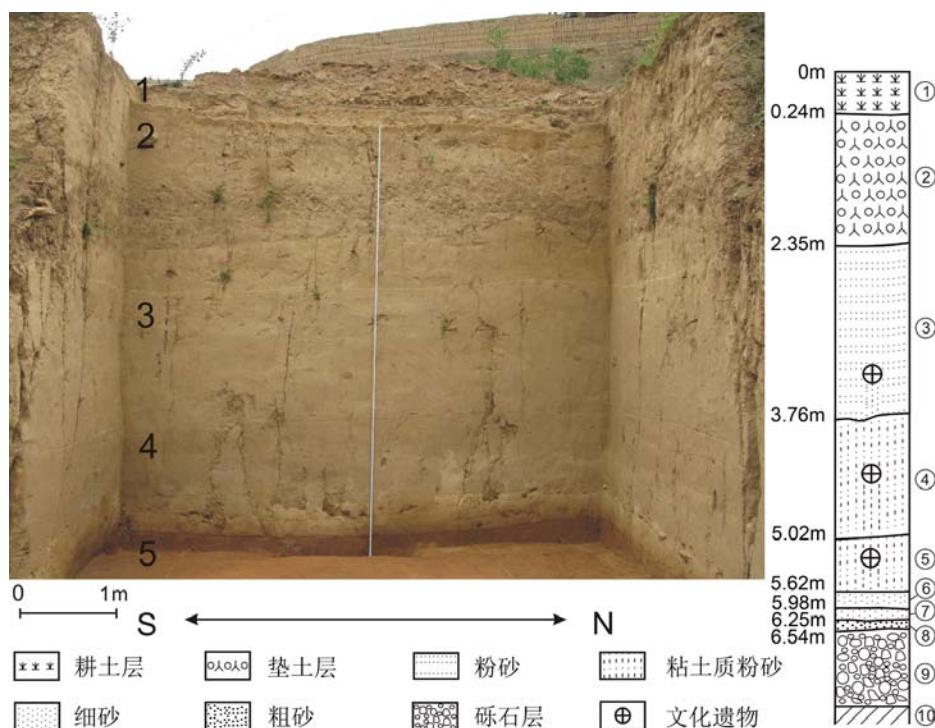
图 4 徐家城遗址地层剖面示意图
