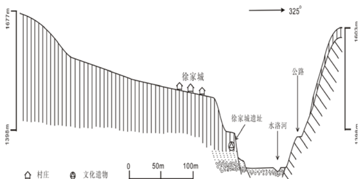
图 2 徐家城遗址地貌位置
