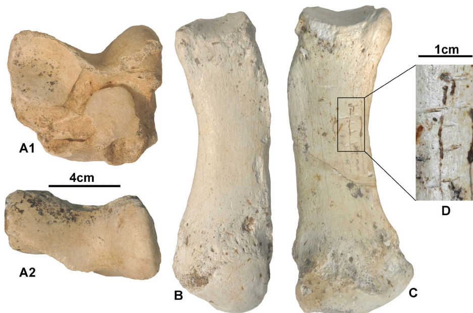
图 4 梅氏犀距骨和掌骨
