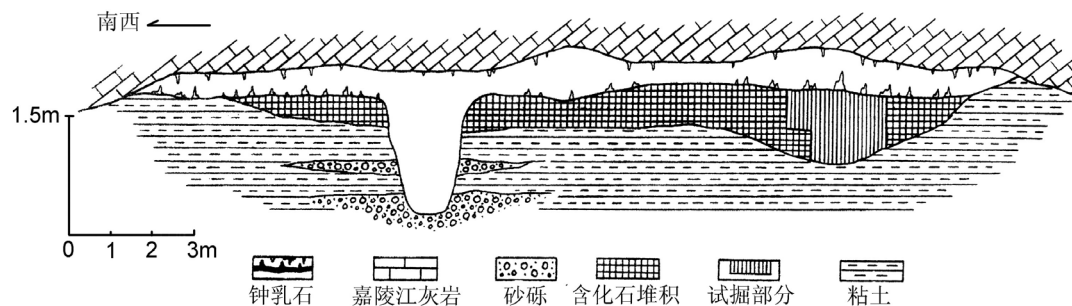
图 1 迷宫洞第 3 地点地质剖面图 [1]
