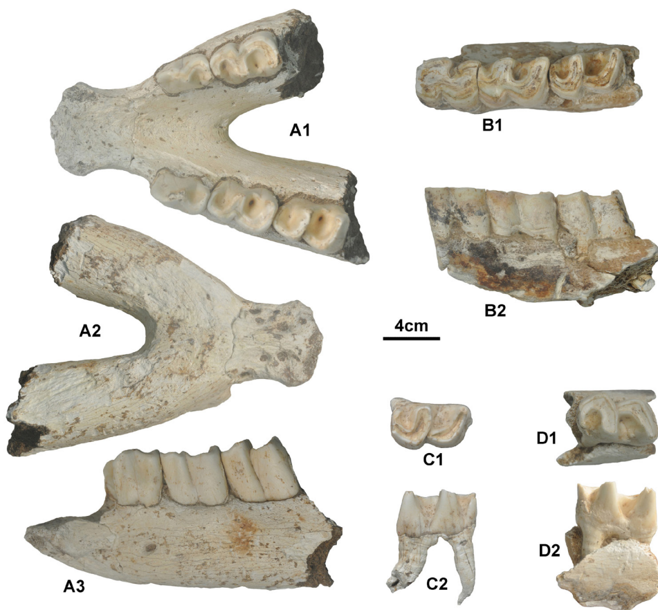
图 2 梅氏犀下颌及下颊齿
