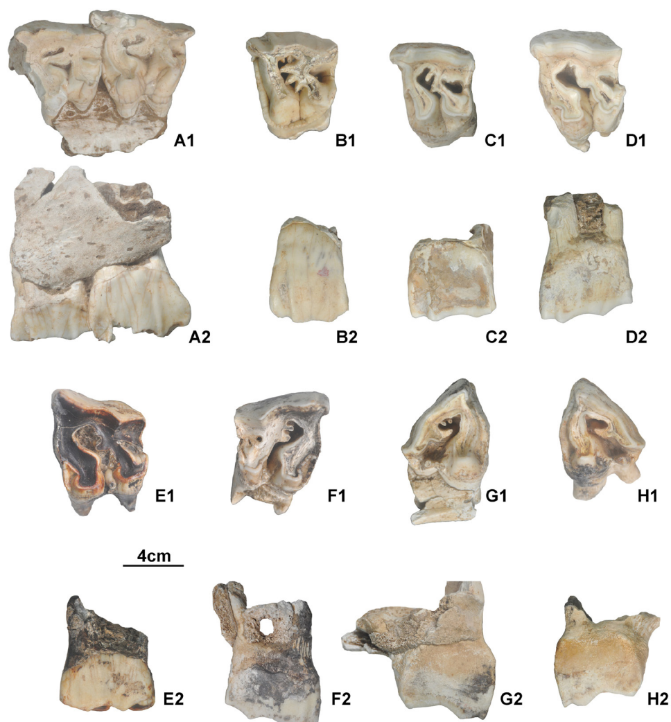
图 3 梅氏犀上颊齿
