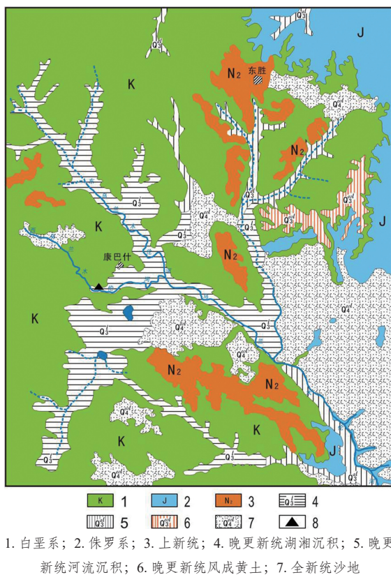
图3 鄂尔多斯新生代地质略图 Fig.3 Cenozoic geological map of Ordos) [22]
