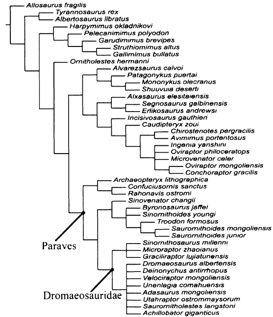
图 4 陆家屯纤细盗龙(新属新种)的系统位置
