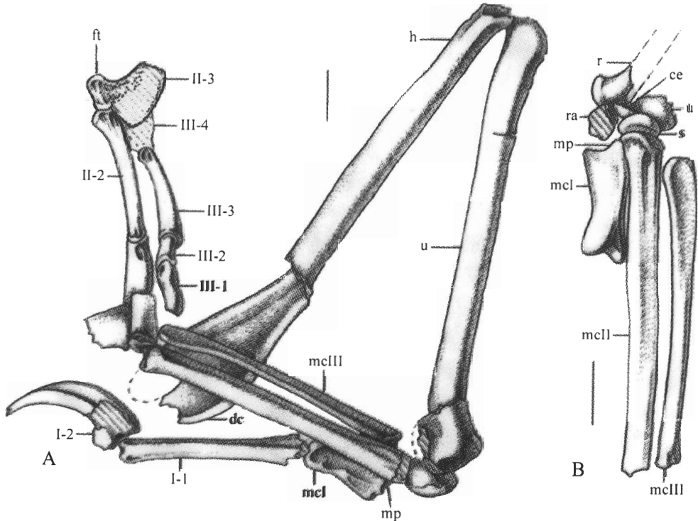
图2 陆家屯纤细盗龙(新属新种)正型标本(IVPP V 13474),比例尺 = 1 cm
